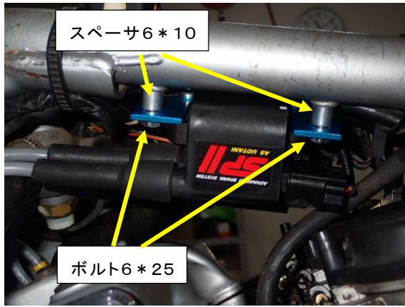
図3、#1&4コイル
