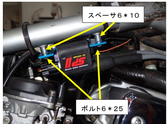
図4、#2&3コイル
