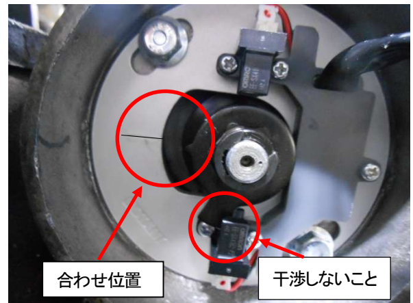
図6、ピックアップASSYの装着 (プレートがなるべく中心になる ように取付けて下さい)
