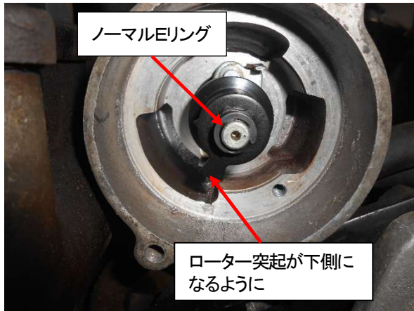
図3、タイミングローターの装着
