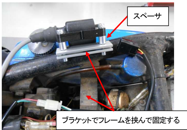
図5、SP2コイルの装着
