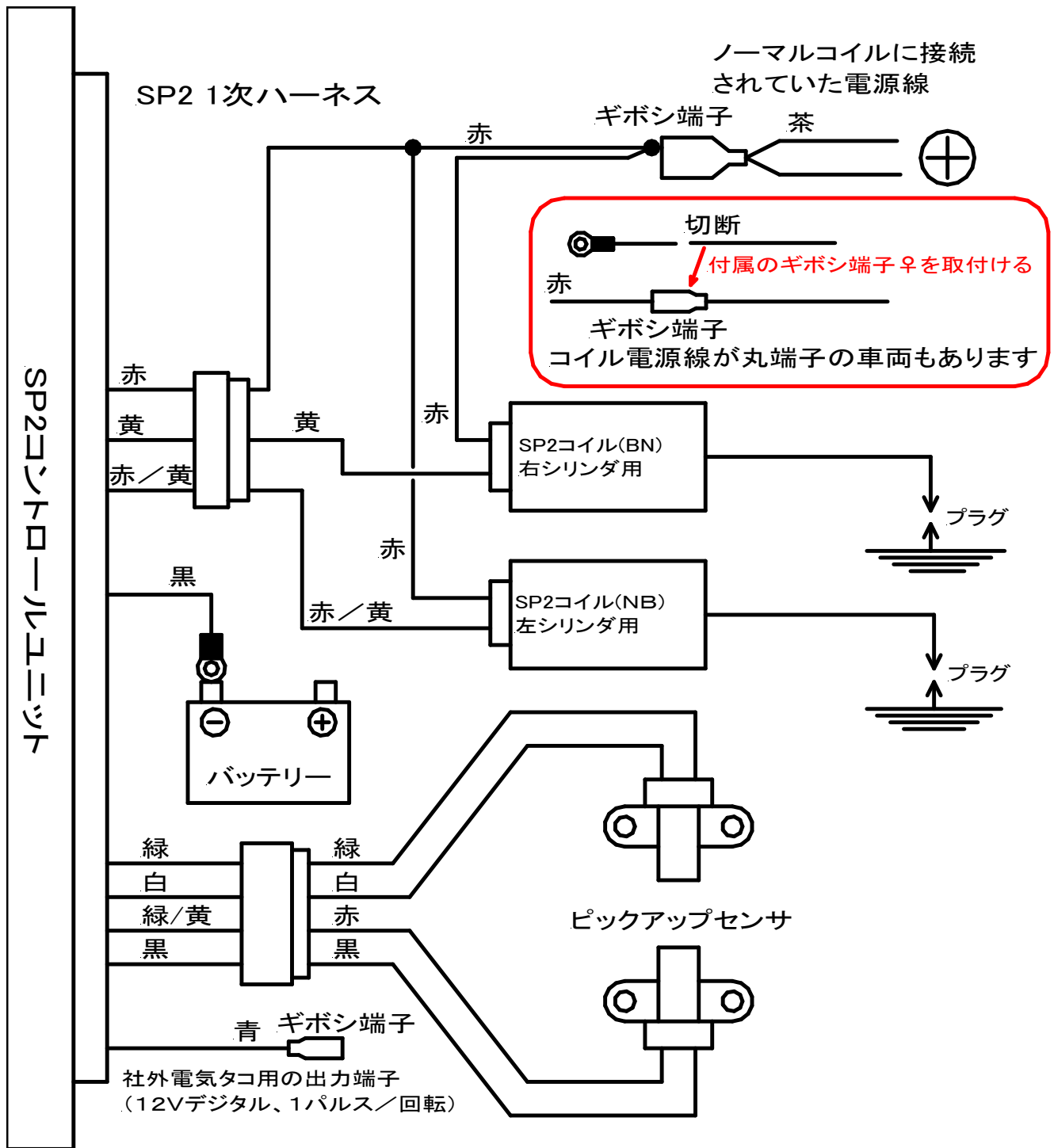
図9、SP2点火システム配線図
