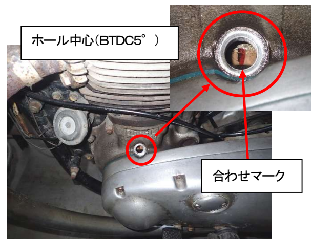
図2、点火時期合わせ位置(右シリンダー一点火点)
