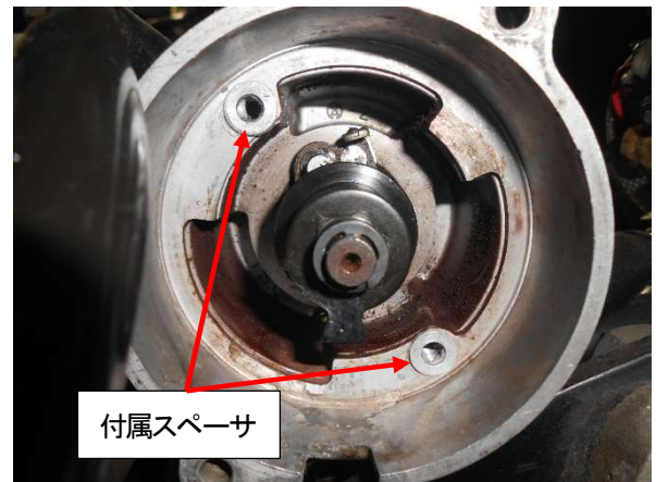
図4、スペーサの貼り付け (W1SA、W3のみ)
