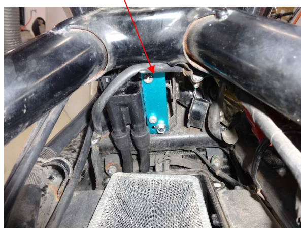
図6、図7、SP II イグニッションコイルの取付け
