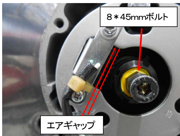
図3、タイミングローターの取付 エアギャップを0, 4~0.6mm に合わせる
