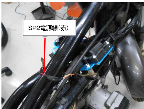
図5、電源接続、ノーマルコイルの電源線に接続(橙/白、左右どちらでも可)
