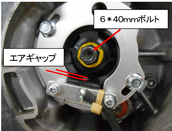
図3、タイミングロータを取付けてエアギャップを0.4~0.6mmに合わせる
