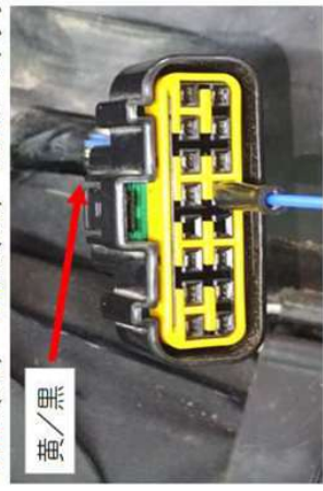
4HME('01)~4HMG('03) 16ピンコネクタ
