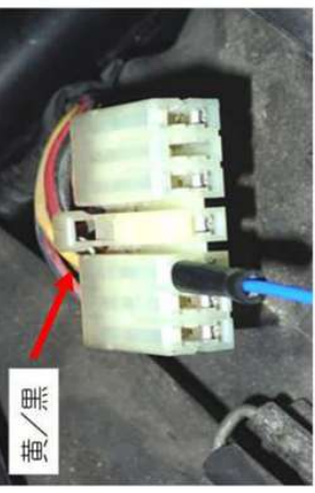
4HM1('93)~4HMD('00) 13ピンコネクタ
