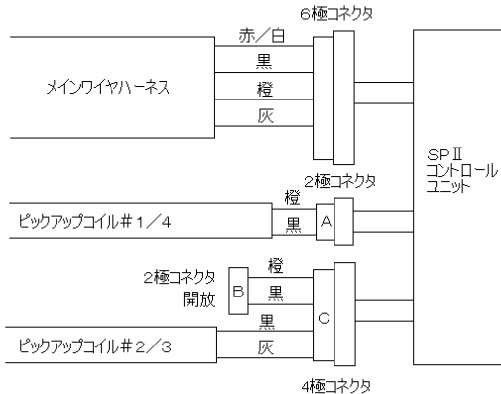
SP IIコントロールユニット 接続図
