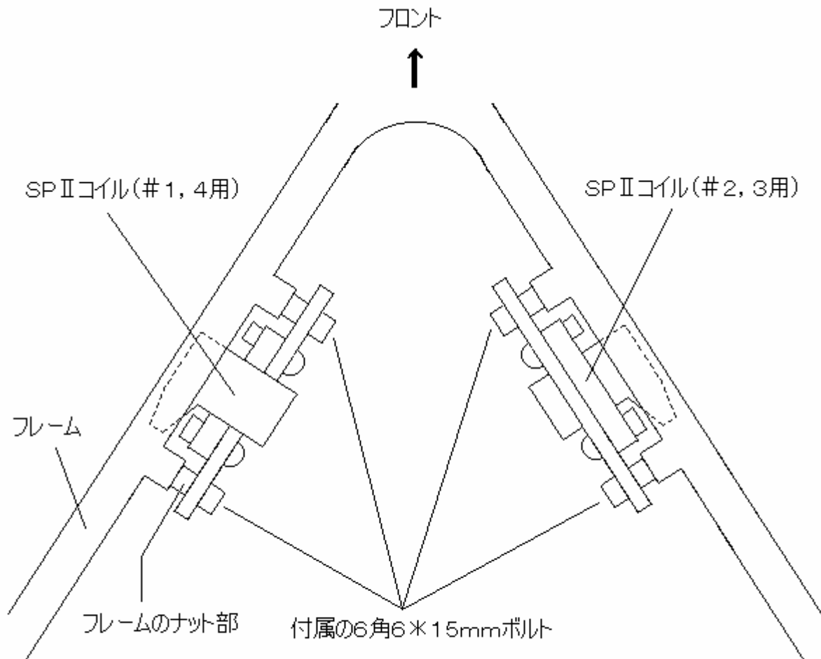
SPⅡコイル装着図(上から見た図)
