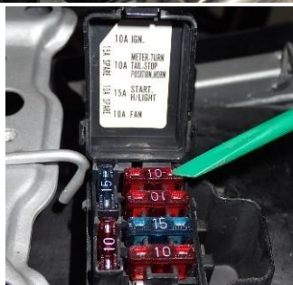
図4 ヒューズ交換 10A→15A
