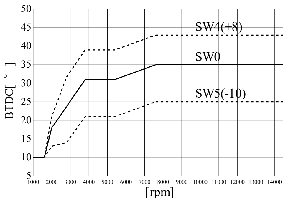
SP2FPKit(H.RVF400) ignition curve
