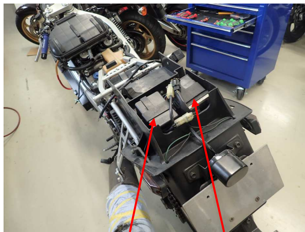
図4、ノーマルCDIコンバータ/コントローラを外す
