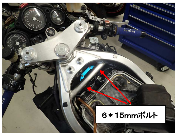
図2、SP II コイル(2・4フロント用)の取付
