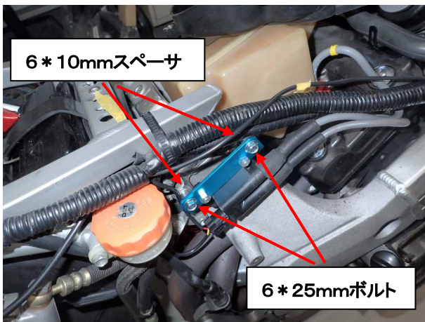
図3、SP II コイル(1・3リヤ用)の取付
