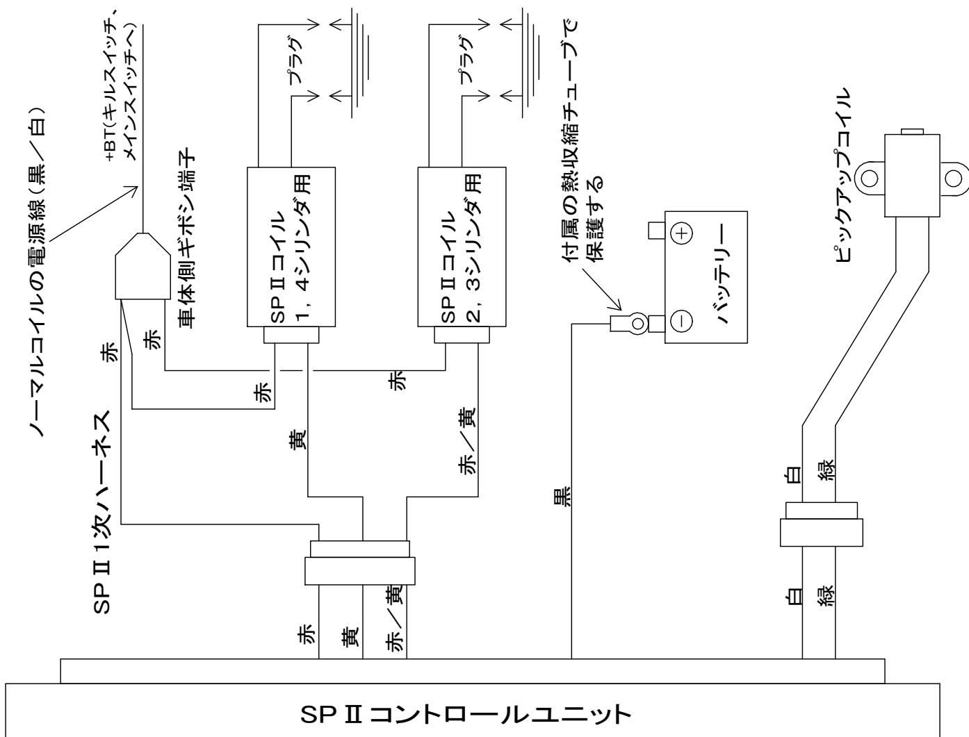
図7、SP II 点火システム配線図
