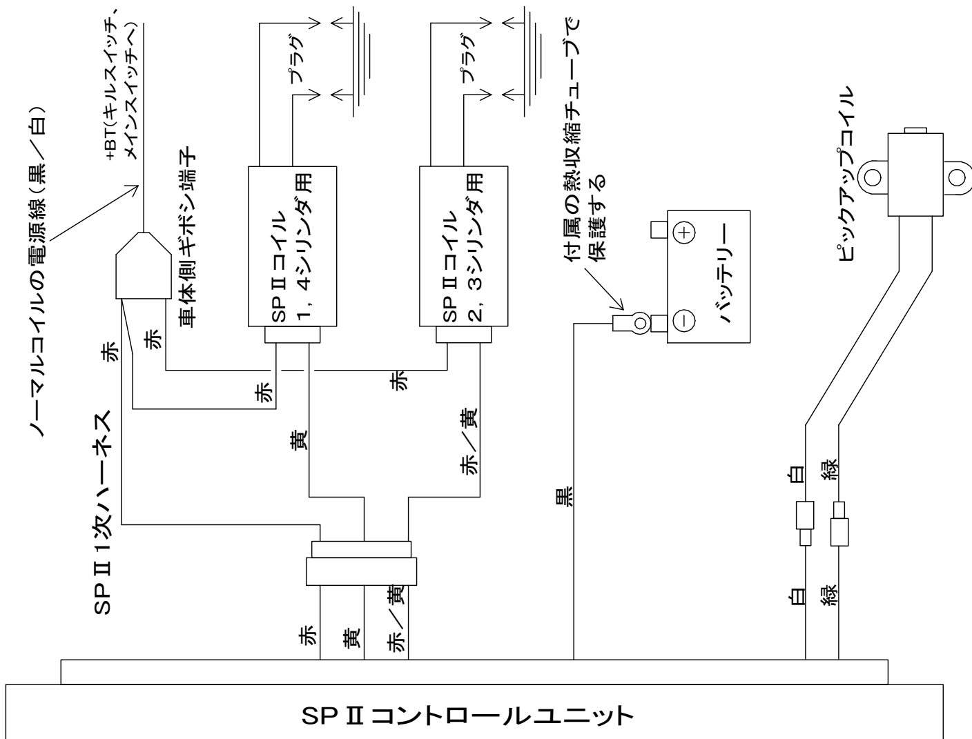
図7、SP II 点火システム配線図
