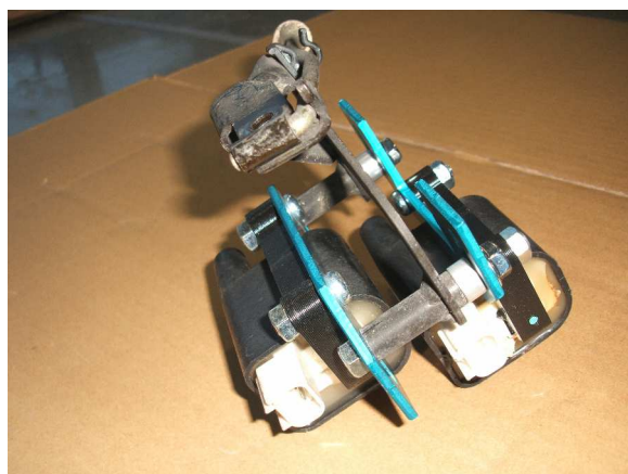
図2、SP II コイル取付(フロントから見た場合) 6 * 50mmボルト、6 * 6mmスペーサ使用。
