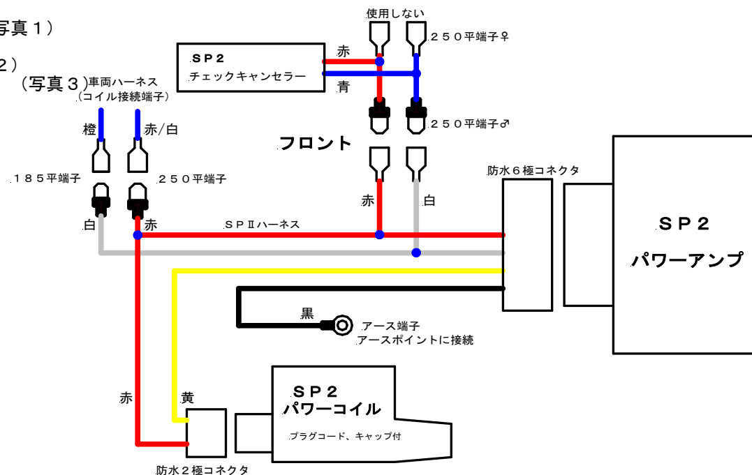
図1 配線図
