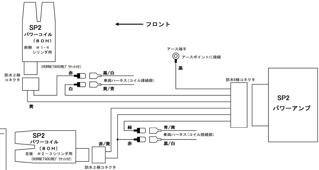
図2 配線図
