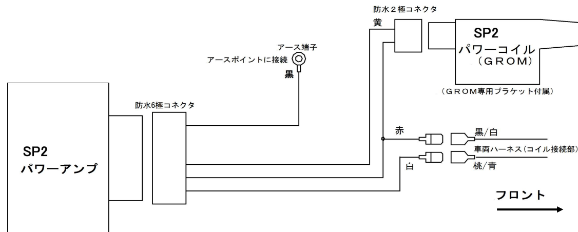
図1配線図
