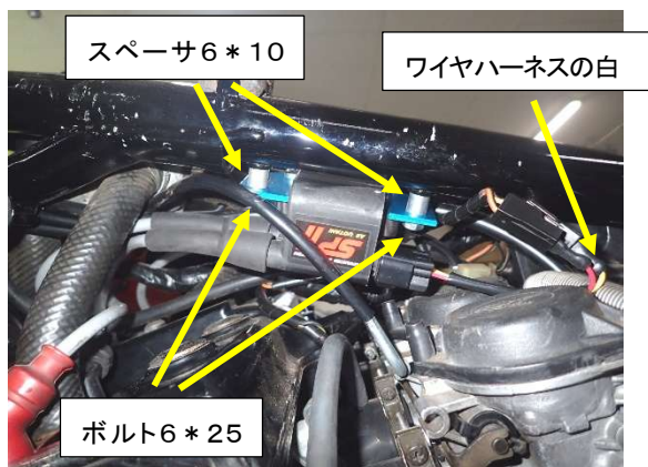
図3、#1&4コイル
