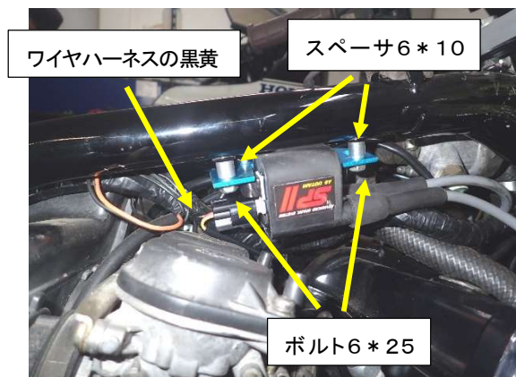
図4、#2&3コイル
