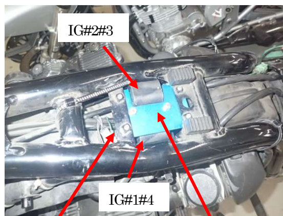
図4、 SP2 コイルの取り付け
