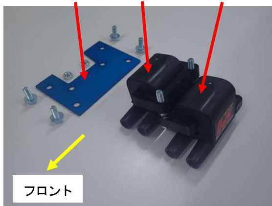
図3、 ブラケット コイル(2P) コイル(2P)H
