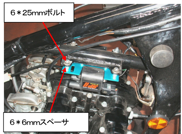
図6、SP2 コイルの装着
