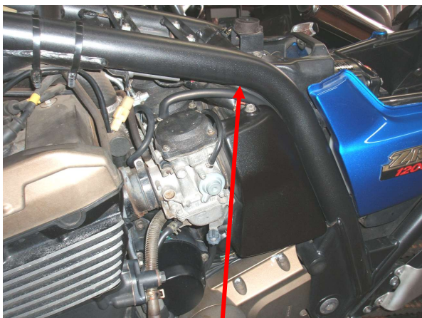
図3、パルシングコイルのコネクタ(2極T型、黒)
