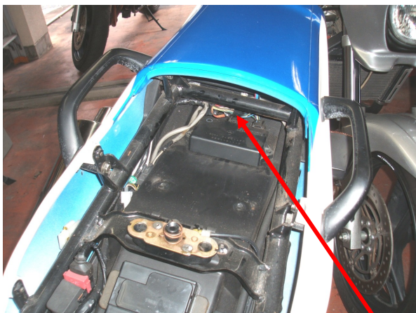
図1、ノーマルイグナイタを取外す
