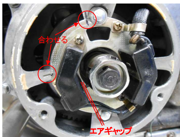
図4 パルスジェネレーターの取付 位置、エアギャップの確認調整 (0.4~0.6mm)
