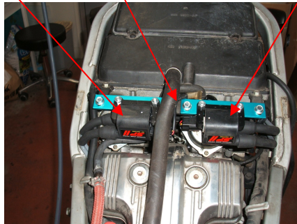
図2、SP2コイルの装着
