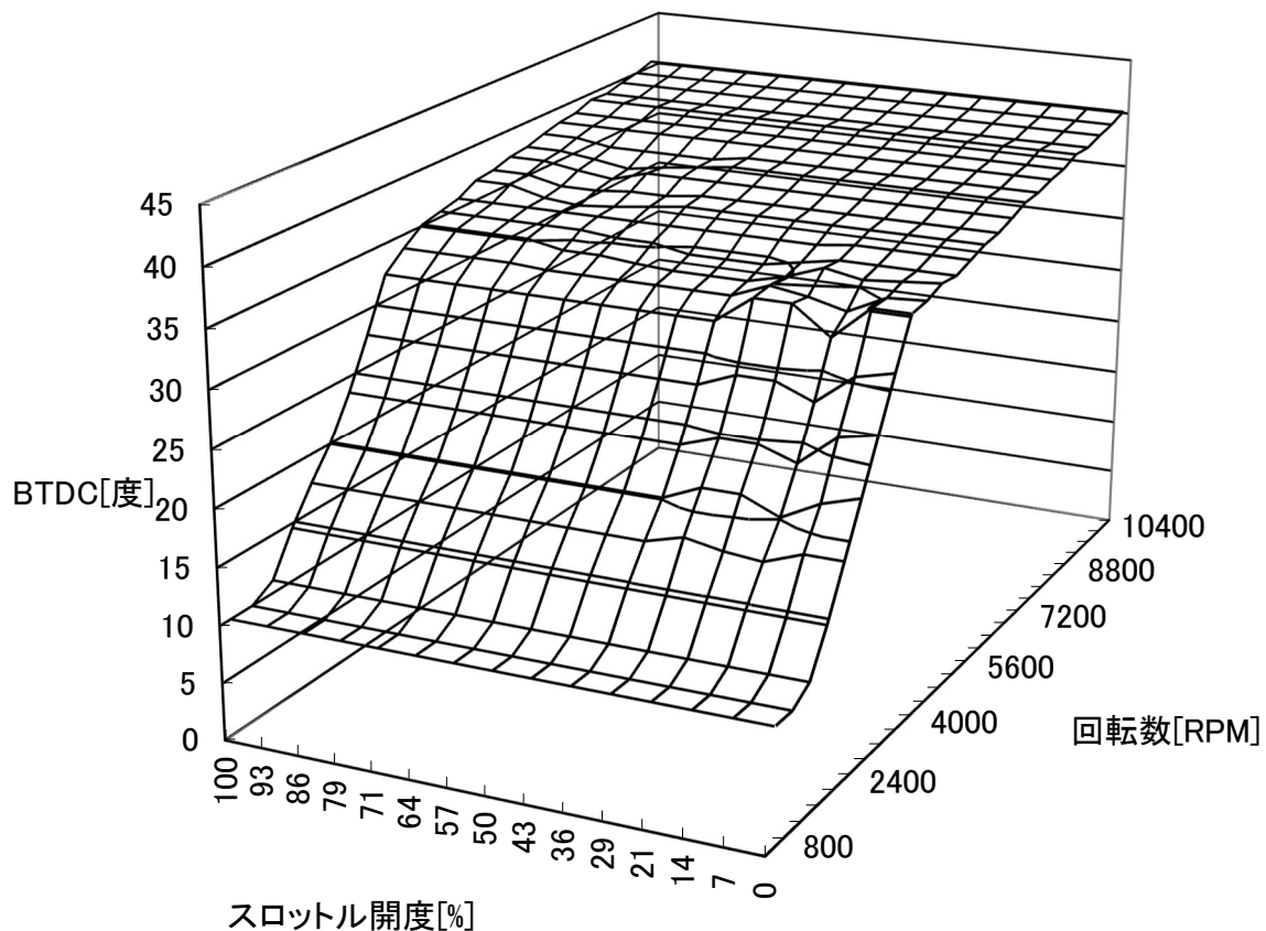
SP2点火マップ(0マップ) H.CB750
